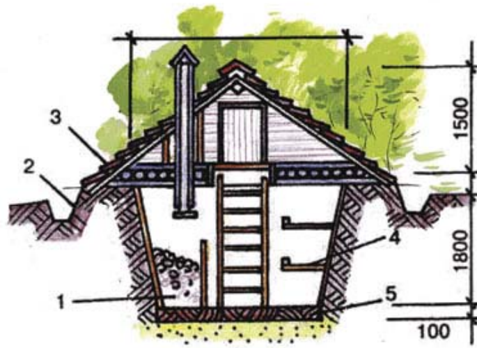
Рис. 8. Заглиблений льох: 1 – овочеві засіки, 2 – водовідведення, 3 – дах, 4 – полиці, 5 – підлога;
