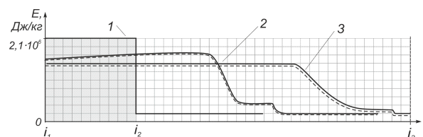
Рис. 5. Результаты численного моделирования влияние теплообмена со стенкой канала: 1, 2, 3 – удельная полная энергия газового потока на момент времени 0; 3,1; 7,1 мс; сплошная линия \alpha = 0\ \text{Вт}/(\text{м}^2\cdot\text{К}) , штриховая линия – \alpha = 10\ 000\ \text{Вт}/(\text{м}^2\cdot\text{К}) / Fig. 5. The results of numerical simulation of the effect of heat exchange with the channel wall: 1, 2, 3 – specific energy flow of gas at time 0; 3,1; 7,1 ms; solid line \alpha = 0\ \text{W}/(\text{m}^2\cdot\text{K}) , dashed line – \alpha = 10\ 000\ \text{W}/(\text{m}^2\cdot\text{K})
