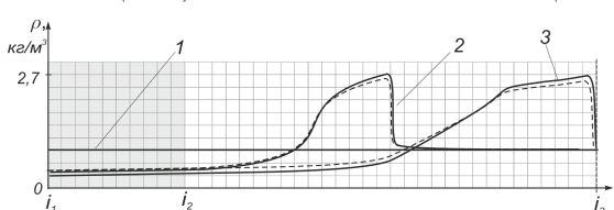
Рис. 4. Результаты численного моделирования влияние теплообмена со стенкой канала: 1, 2, 3 – плотность газового потока на момент времени 0; 3,1; 7,1 мс; сплошная линия \alpha = 0\ \text{Вт}/(\text{м}^2\cdot\text{К}) , штриховая линия – \alpha = 10\ 000\ \text{Вт}/(\text{м}^2\cdot\text{К}) / Fig. 4. The results of numerical simulation of the effect of heat exchange with the channel wall: 1, 2, 3 – gas flow density at time 0; 3,1; 7,1 ms; solid line \alpha = 0\ \text{W}/(\text{m}^2\cdot\text{K}) , dashed line – \alpha = 10\ 000\ \text{W}/(\text{m}^2\cdot\text{K})
