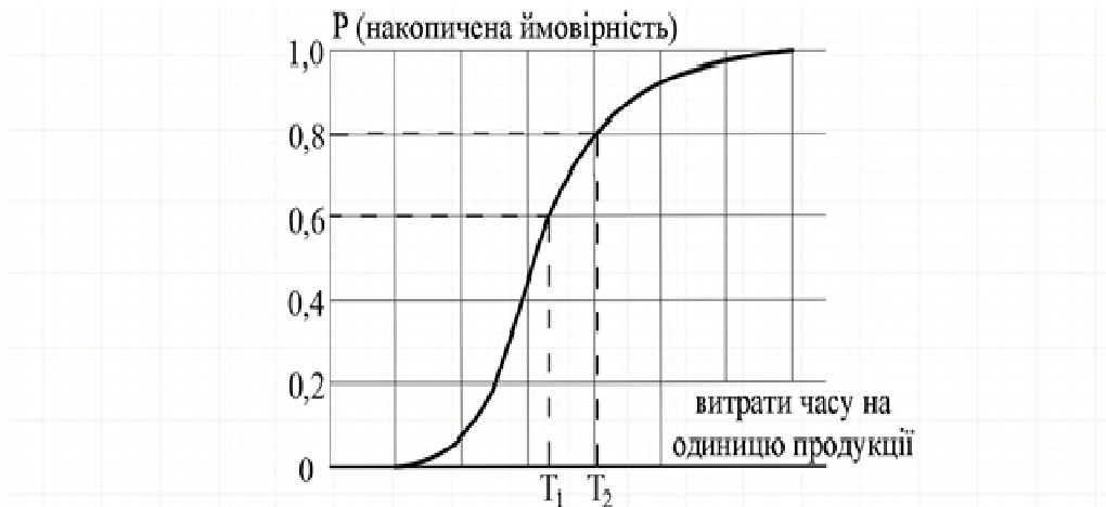
Рис. 1. Підсумкова функція часу закінчення робіт із визначенням тривалостей робіт за надійності 60 і 80 % / Fig. 1. The final function of the completion time of work with the definition of the duration of work for the reliability of 60 and 80 %
