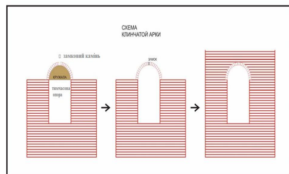
Рис. 12. Схеми клинчастої арки / Fig. 12. Scheme of wedge arches
