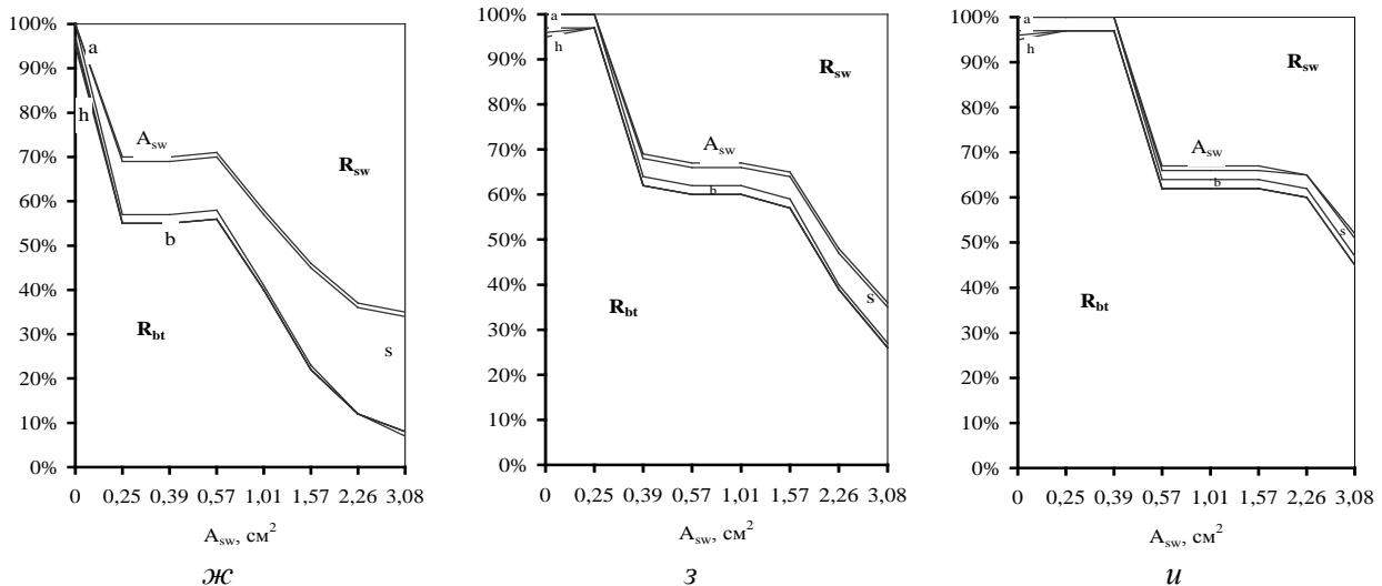
Рис. 3. Ранжування параметрів залізобетонних елементів, що згинаються, за критерієм внеску в дисперсію міцності похилих перерізів: крок поперечної арматури а, з, ж – 5 см; б, д, з – 10 см; в, е, и – 15 см; при розрахунку за варіантами: а, б, в – першим; г, д, е – другим; ж, з, и – третім
