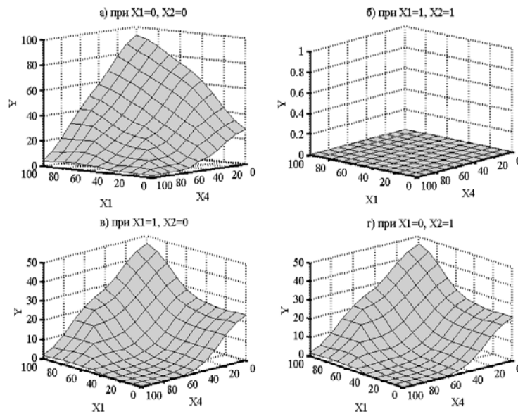
Рис. 1. Поверхні «входи – вихід» нечіткої моделі до реалізації етапу параметричної ідентифікації
