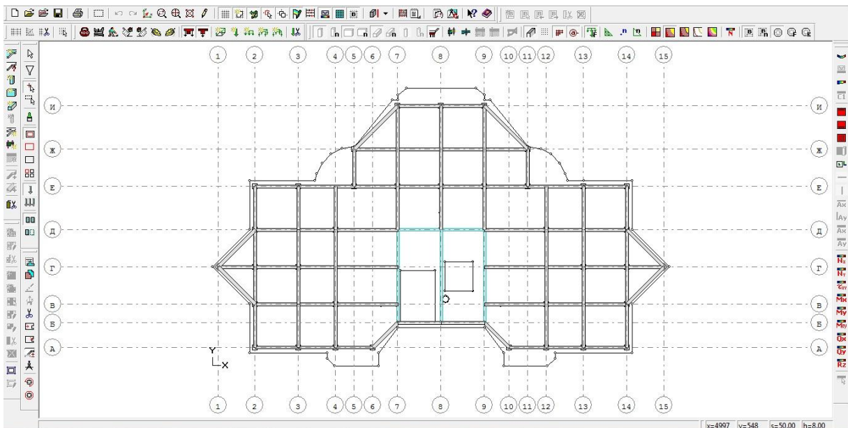
Рис. 2. Ребристе перекриття з плитами, опертими по контуру
